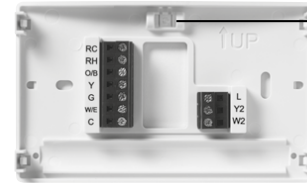
Nivelación del termostato La nivelación es solo por razones estéticas y no afectará el funcionamiento del termostato.
