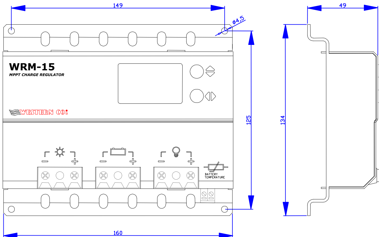
Fig. 8 Dimensions
