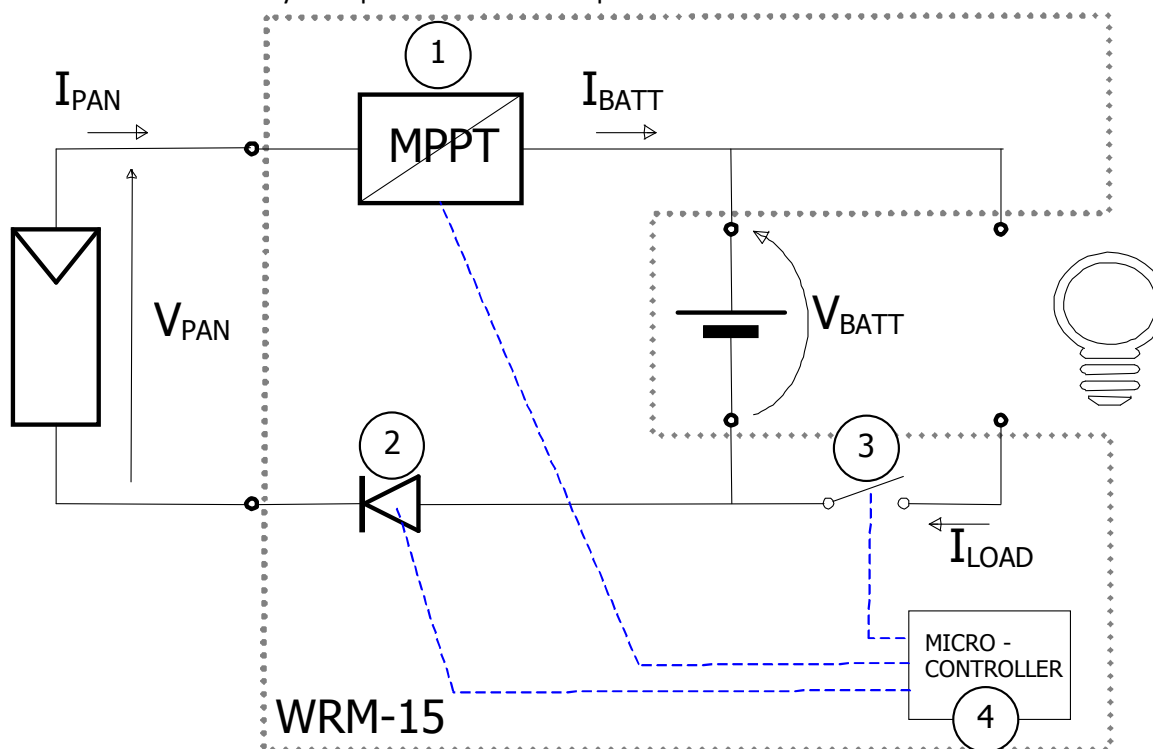
Fig. 1 schematic
